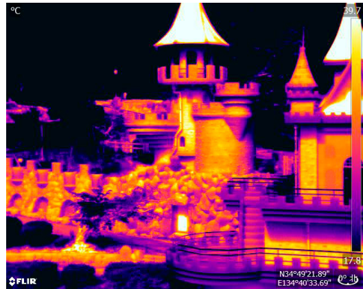
ZENMUSE XT2 で撮影した赤外線画像。温度差を測定することにより、外壁タイルの浮き等を検出することができる。
